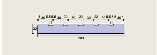
プレキャスト製品P-1型の断面図
