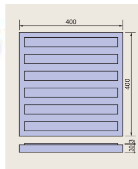
線状・T-10 ゴム入テラゾー製品 幅300×長300×厚30m/m(5条) 幅400×長400×厚30m/m(6条)
