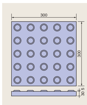
点状・T-4(25点) プレキャスト製品 幅300×長300×厚30m/m
