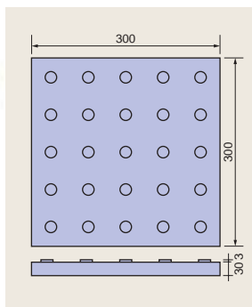
点状・T-9 ゴム入テラゾー製品 幅300×長300×厚30m/m(25点) 幅400×長400×厚30m/m(36点)
