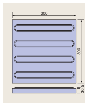
線状・T-2(4条) プレキャスト製品 幅300×長300×厚30m/m
