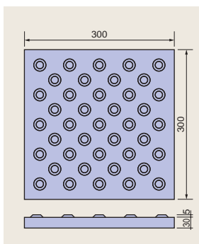
点状・T-7(41点) プレキャスト製品 幅300×長300×厚30m/m
