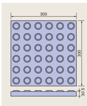
点状・T-1B(36点) プレキャスト製品 幅300×長300×厚30m/m
