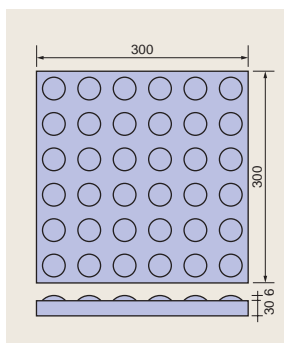
点状・T-1A(36点) プレキャスト製品 幅300×長300×厚30m/m
