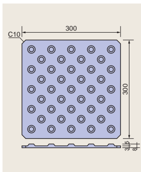
点状・N-1 合成ゴム製品 幅300×長300×厚8m/m
