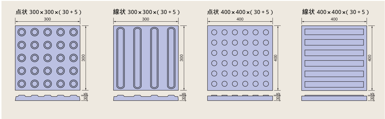
幅300×長300×厚(30+5)m/m
